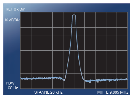
600-Hz-Roofing-Filter (9 MHz, SPANNE: 20 kHz)
