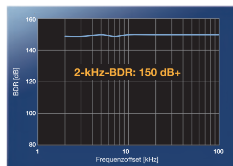
14-MHz-Band-Sperre Dynamischer Bereich (BDR)
