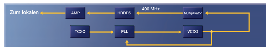
Blockdiagramm lokaler Stromkreis
