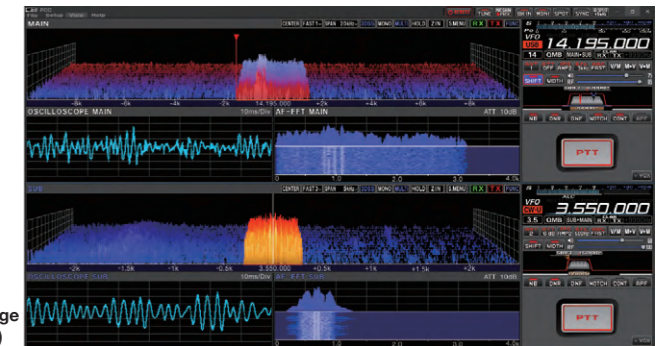
Wasserfallanzeige (MONO)
