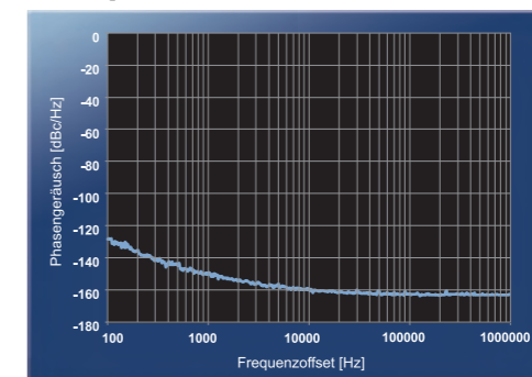
1. lokaler OSZ Phasengeräusch (14.2 MHz)
