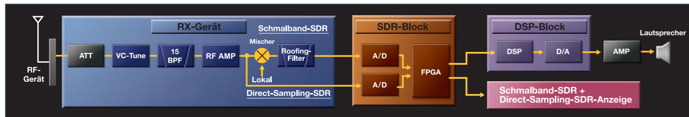
Hybrid-SDR-Konfiguration
