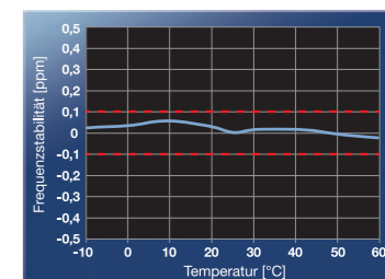
TCXO-Stabilität gegen Temperatur
